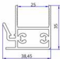
PG010 - COPERCHIO GUIDA GHIGLIOTTINA RIF:37270
