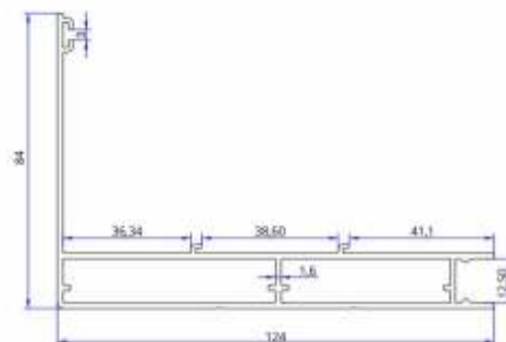
PG006 - TELAIO INFERIORE GHIGLIOTTINA RIF:37263
